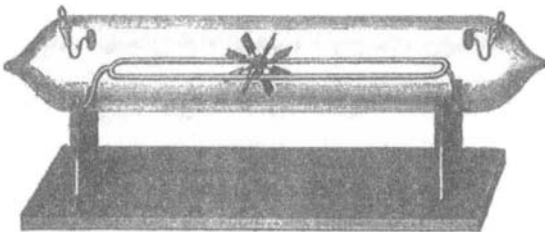
أنايب كروكس: أشعة الكاثود تضيء ماسة، وتعكس ظلاً لصليب مالطي، وتحرك دولاب تجديف صغيراً
