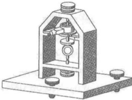
رسم مايكلسون لمرآته الدوارة
