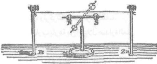
تجربة أورستد
