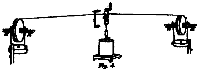
النسخة المنقحة من تجربة جول
